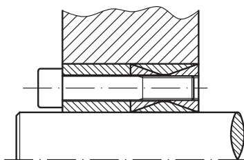
Fijación de un cubo mediante un TEK-200 con anillo centrador especial.
